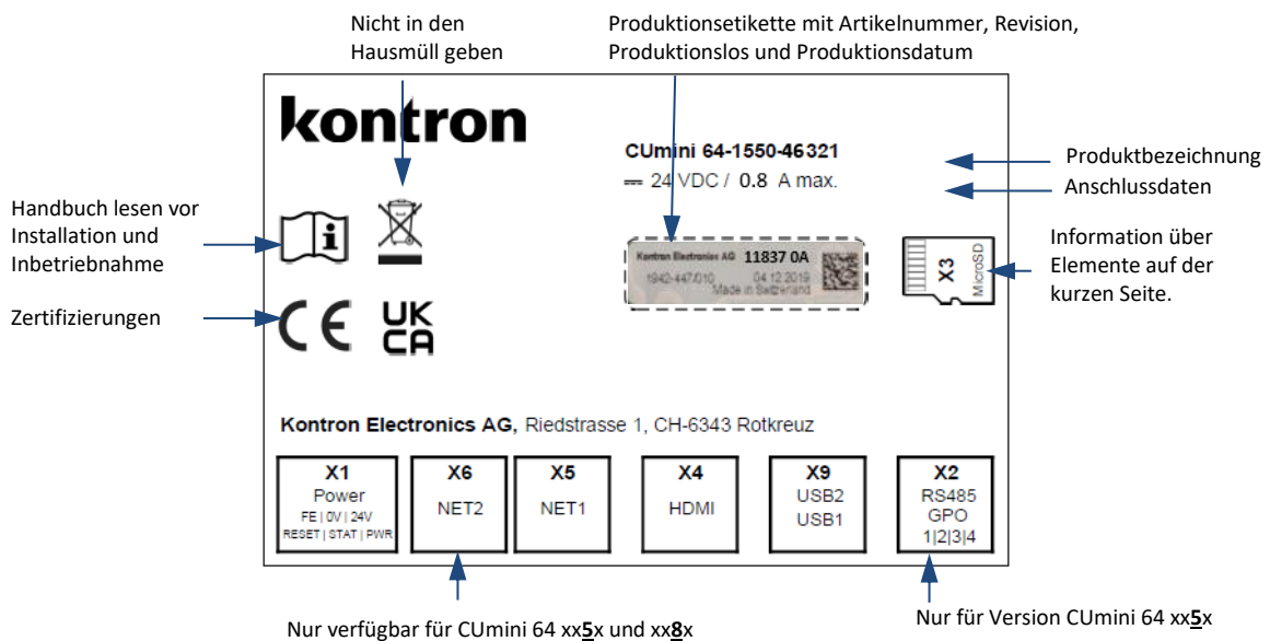
Abbildung 1: Typenschild und Produktkennzeichnung
