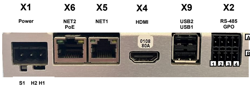
Abbildung 3: Schnittstellen - Ansicht von vorne
