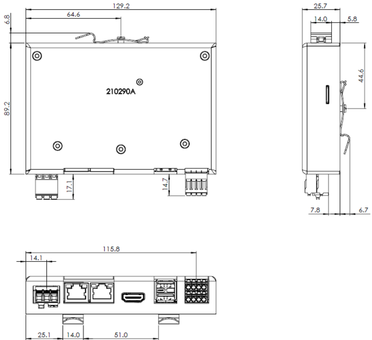
Abbildung 6: Technische Zeichnungen CUmini 6x
