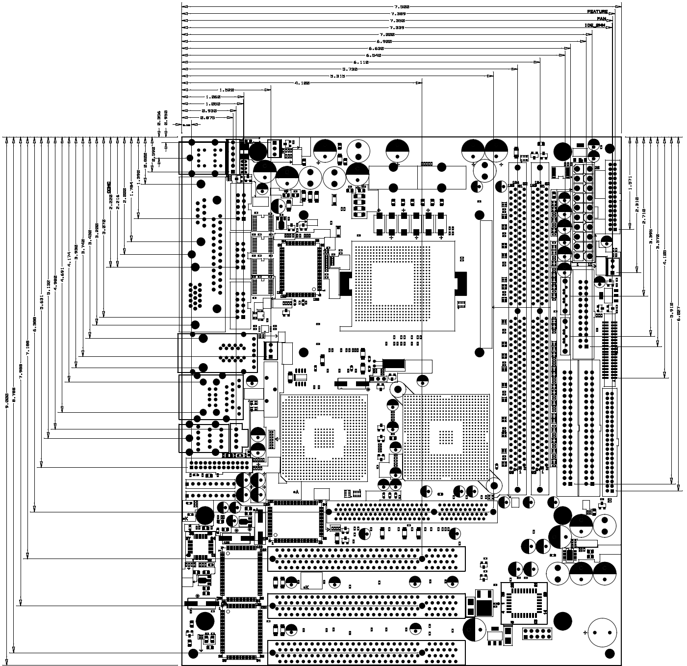
SILKSCREEN_TOP
